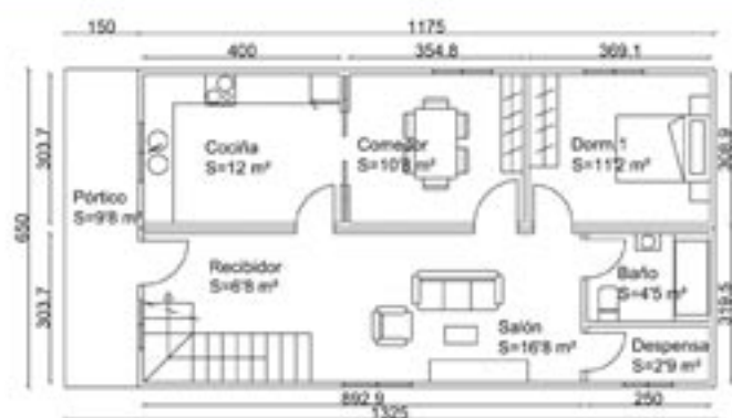
PLANTA BAIXA
