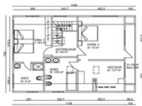
PLANTA ALTA
