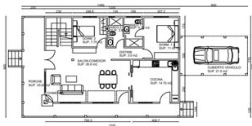
PLANTA BAIXA
