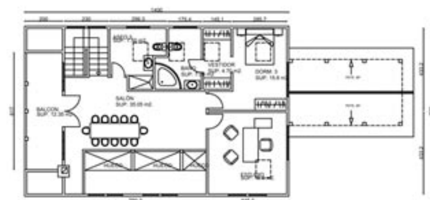
PLANTA ALTA
