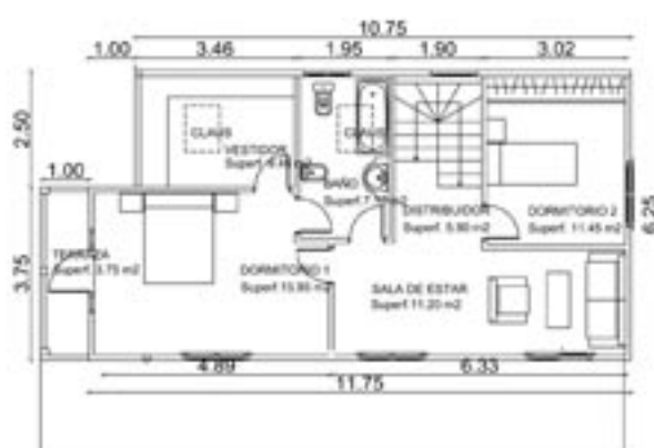
PLANTA ALTA
