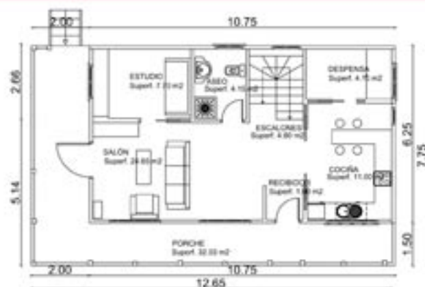
PLANTA BAIXA
